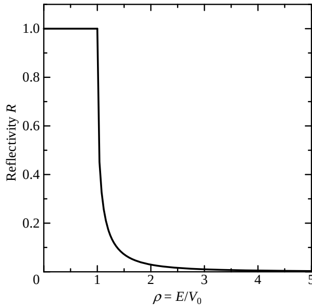
図 10 高さ V_0 のポテンシャル障壁における自由粒子（エネルギー E ）の反射率
