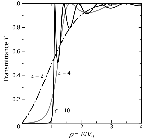
図 12 障壁を通過するトンネル確率。横軸は入射粒子のエネルギーと障壁高さの比。障壁の高さと厚さを表す \varepsilon = \frac{\sqrt{2mV_0}a}{\hbar} をパラメータとしてプロットしてある。
