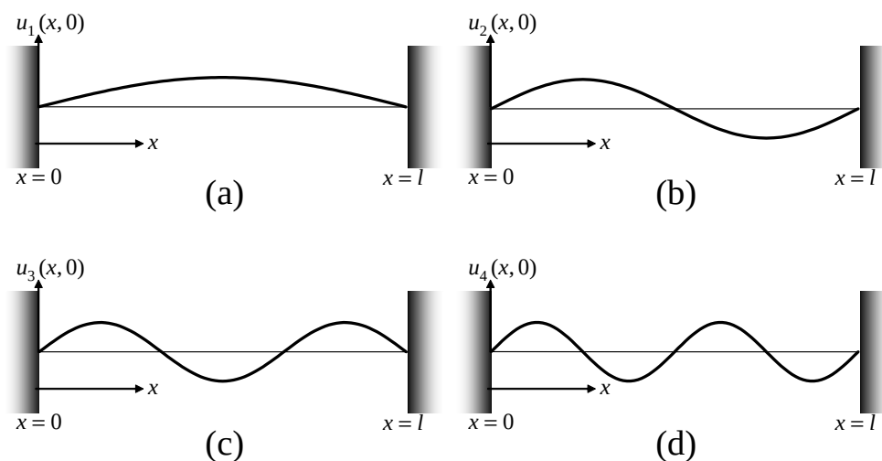
図 4 振動する弦の基準モード。(a) は第 1 調和振動（基本モード）、(b) は第 2 調和振動（第 2 高調波）、(c) は第 3 調和振動（第 3 高調波）、(d) は第 4 調和振動（第 4 高調波）に対応する。
