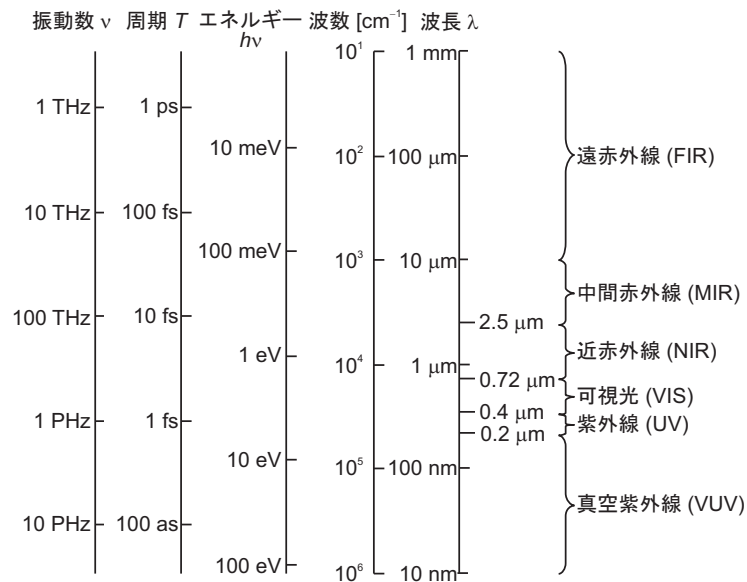
図 19 電磁波と光の分類
