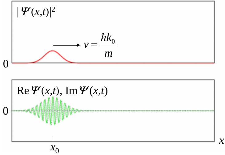
図8 ガウス波束の t = 0 における波動関数と確率振幅
