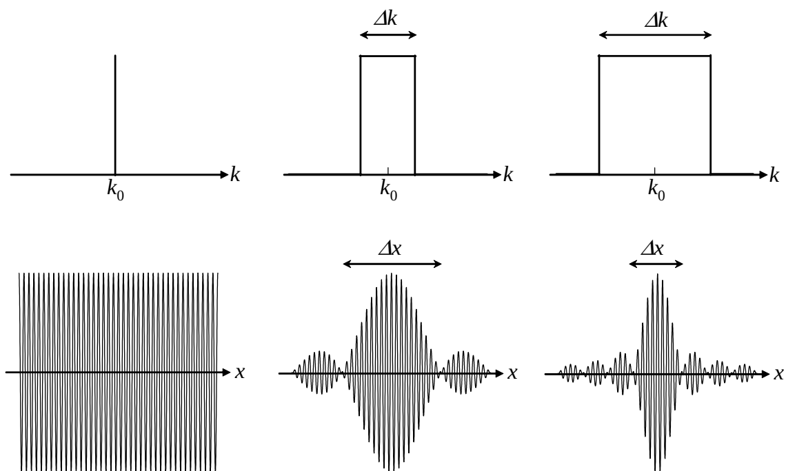
図5 波束のスペクトル F_c(k) (上) とそれに対応する空間波形 f(x) = \int_0^\infty dk F_c(k) \cos(kx) (下)
