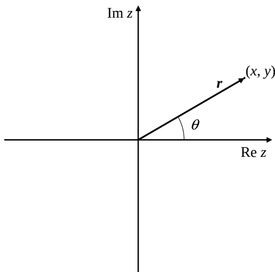
図 7 複素平面と複素数
