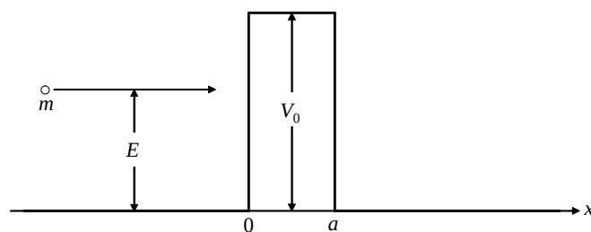
図 11 質量 m エネルギー E の粒子が、高さ V_0 厚さ a のポテンシャル障壁に左から入射する。
