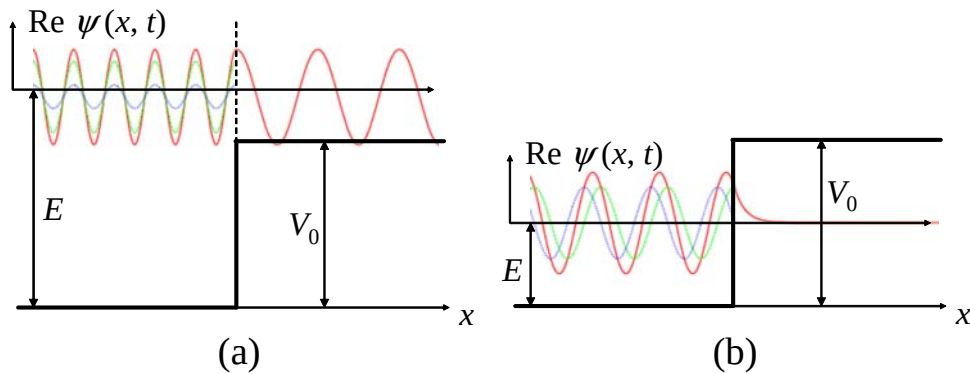
図9 ポテンシャル障壁（高さ V_0 ）によるエネルギー E の自由粒子の反射。(a) は E > V_0 の場合、(b) は E < V_0 の場合である。
