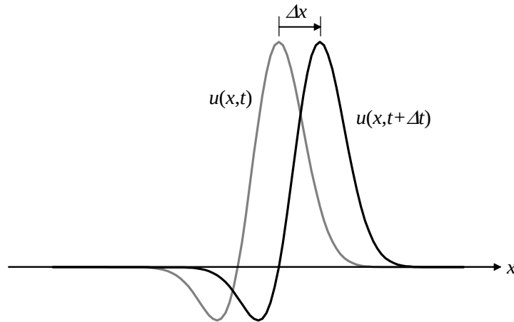
図 2 波動方程式の解 u(x, t) = f(x - vt) の振る舞い。時刻 t と時刻 t + \Delta t における解を示している。
