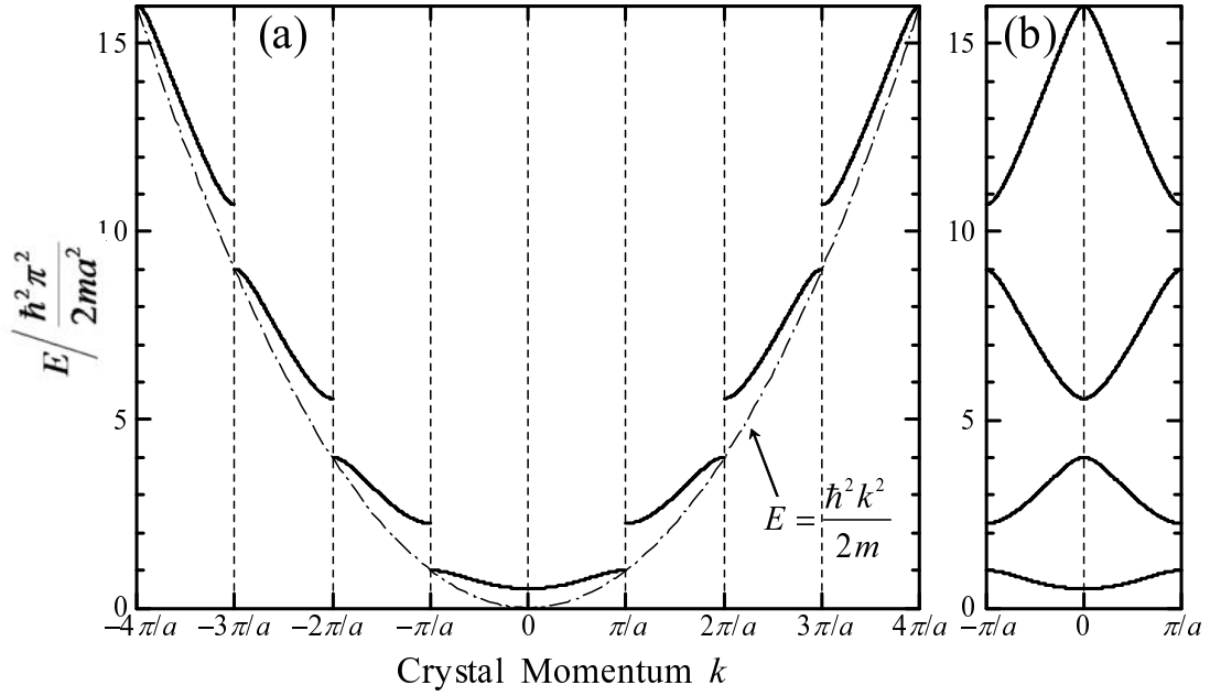
図 17 Kronig-Penney ポテンシャル ( \gamma = 3\pi/2 ) 中の電子の分散関係。(a) は拡張ゾーン形式、(b) は還元ゾーン形式でプロットした。(a) の一点鎖線は自由電子の分散関係を示している。
