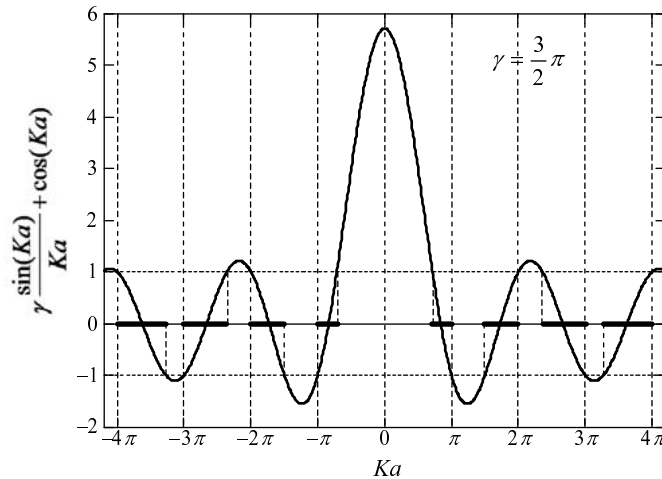
図 16 \gamma = 3\pi/2 の場合の関数 \gamma \frac{\sin(Ka)}{Ka} + \cos(Ka) 。太い実線で示した領域の K の値のみが許される。
