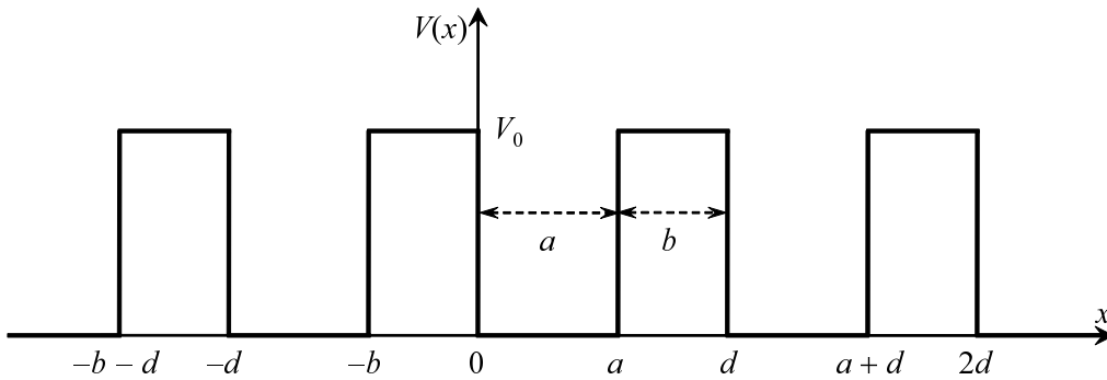
図 15 周期 d の周期ポテンシャル
