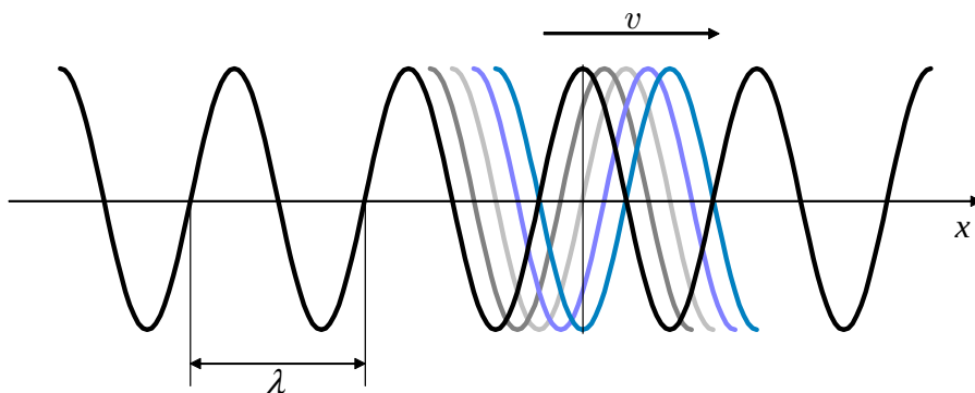
図1 1次元の正弦進行波 A \cos[k(x - vt) + \phi] = A \cos(kx - \omega t + \phi) の振る舞い
