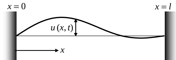
図 3 両端 ( x = 0, l ) を固定した弦の振動
