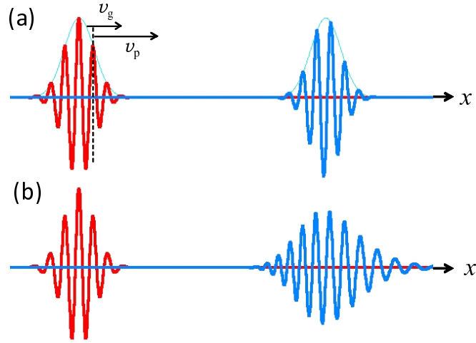
図6 分散性波動の例（ガウス波束）。(a) は群速度分散はないが分散がある場合。波束は形状を変えずに伝搬するが、位相速度と群速度が異なる。(b) は群速度分散もある場合。伝搬に伴い波形が崩れる。パルス広がりやチャーピングが起こっている。
