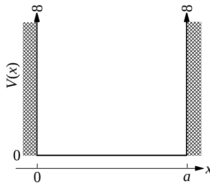
図 13 無限大障壁井戸型ポテンシャル
