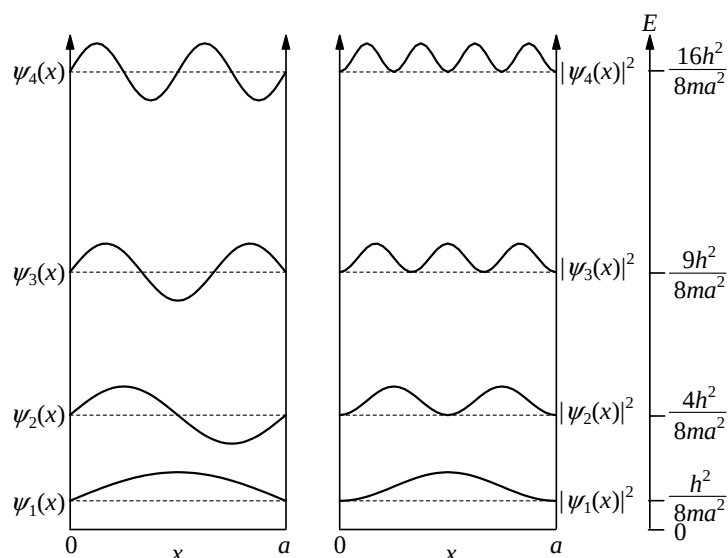
図 14 無限大障壁井戸型ポテンシャル中のエネルギー準位と波動関数 \psi_n(x) (左) および確率密度 |\psi_n(x)|^2 (右)
